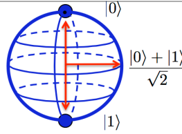
Qubit
